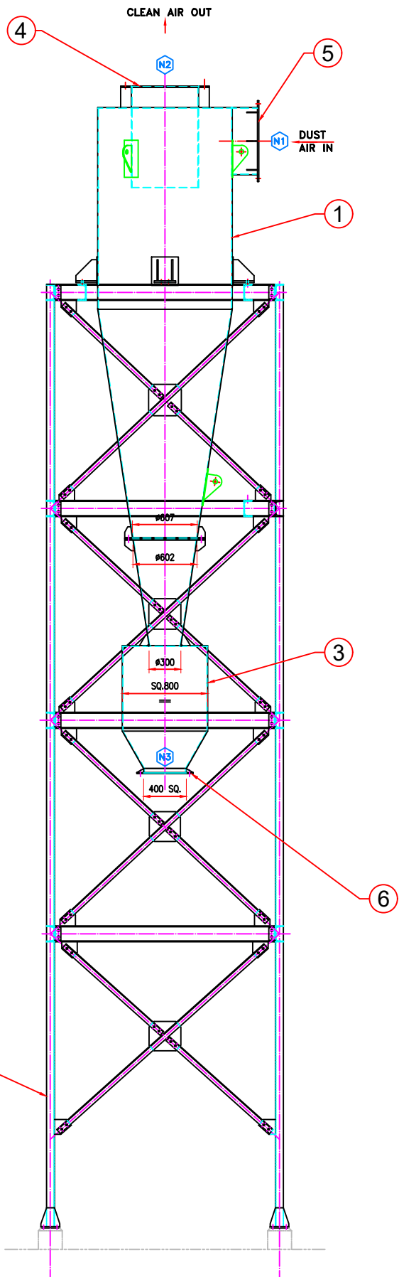
ELEVATION
